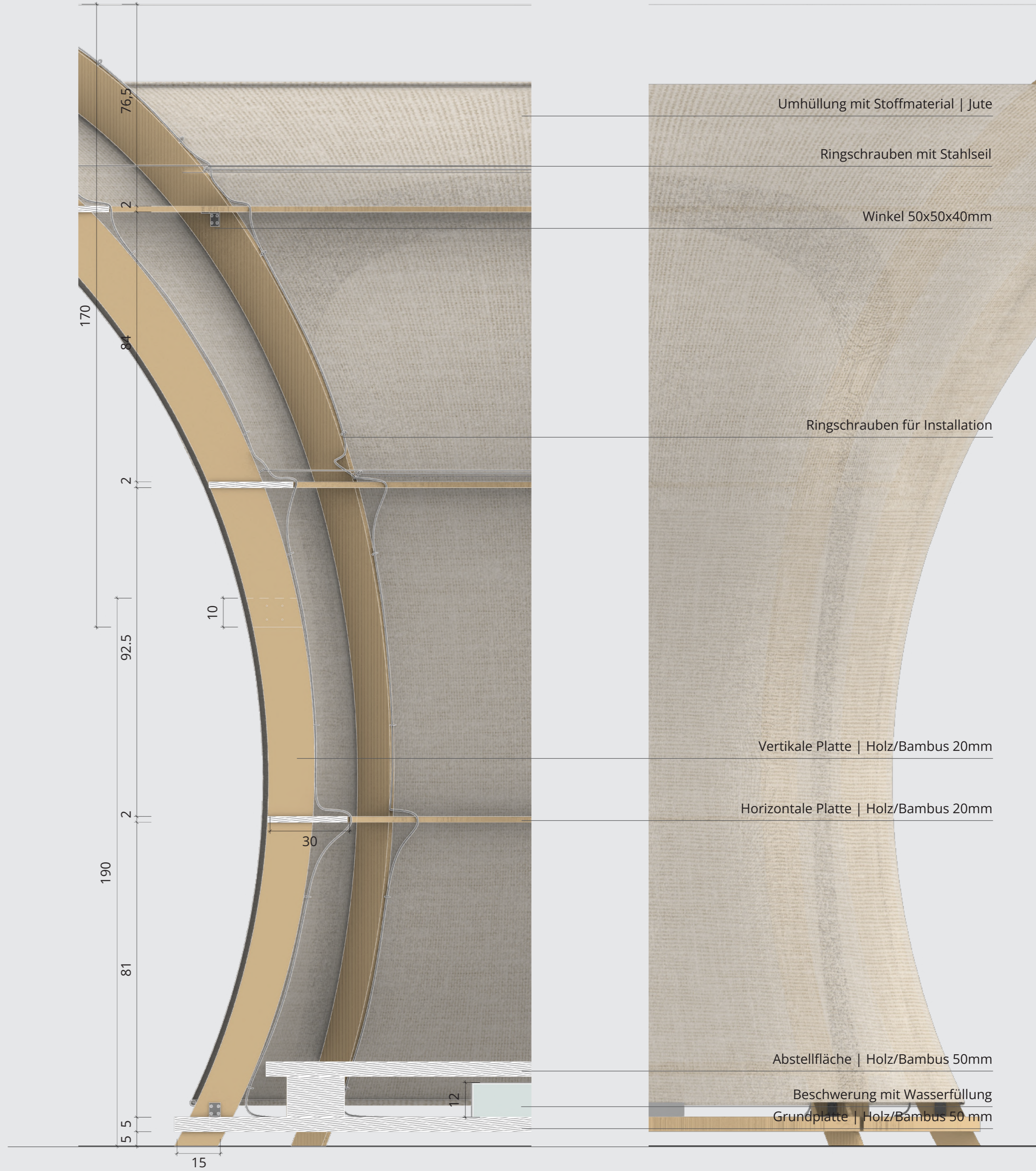
Fassadendetail M 1:10
